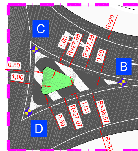
DETALLE "A"
