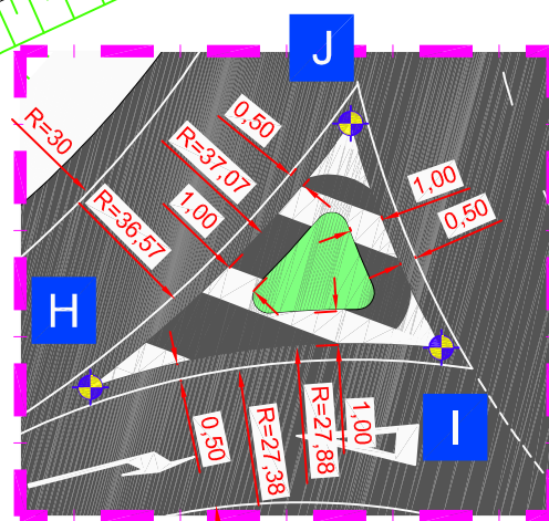
DETALLE "C"
